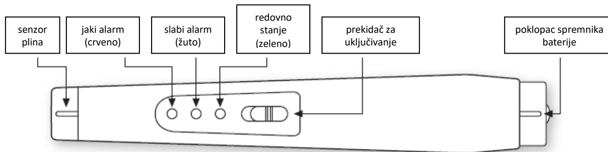
eZsense detektor zapaljivog plina
